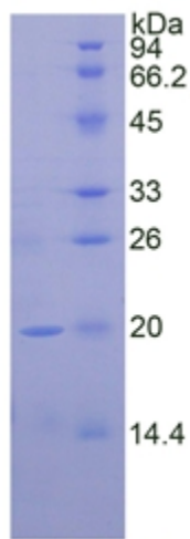
15% SDS-PAGE
