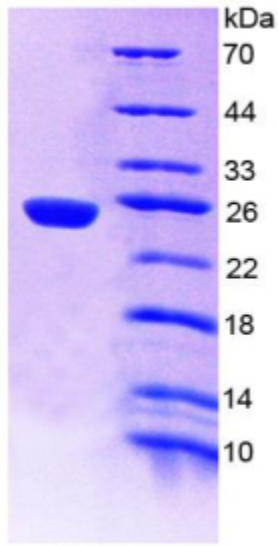
15% SDS-PAGE
