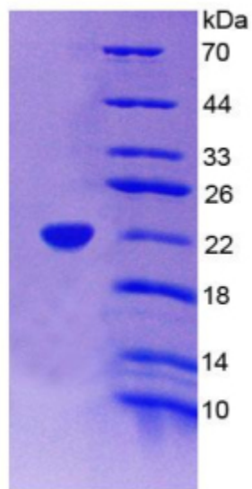
15% SDS-PAGE
