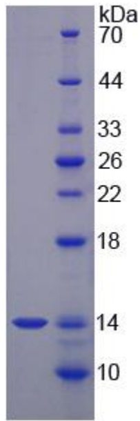
15% SDS-PAGE
