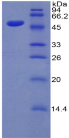
15% SDS-PAGE
