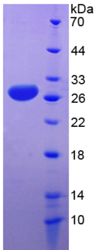
15% SDS-PAGE
