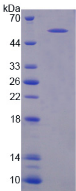
15% SDS-PAGE
