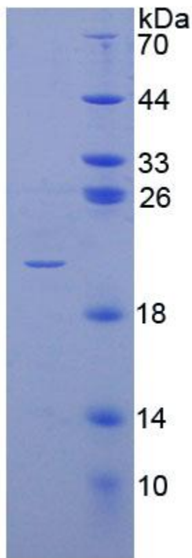
15% SDS-PAGE
