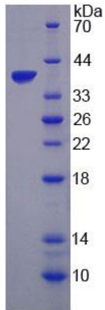
15% SDS-PAGE
