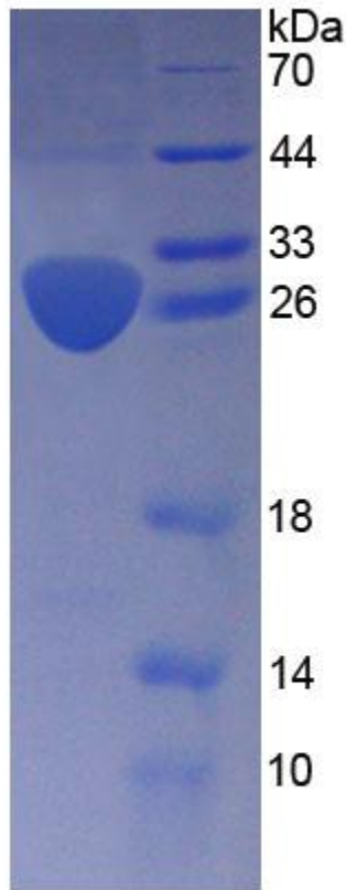
15% SDS-PAGE
