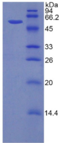
15% SDS-PAGE
