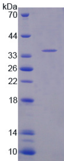
15% SDS-PAGE
