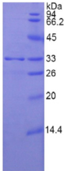
15% SDS-PAGE
