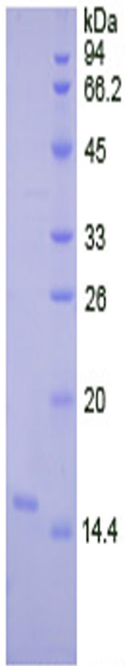
15% SDS-PAGE
