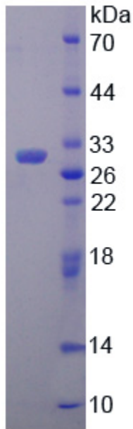
15% SDS-PAGE
