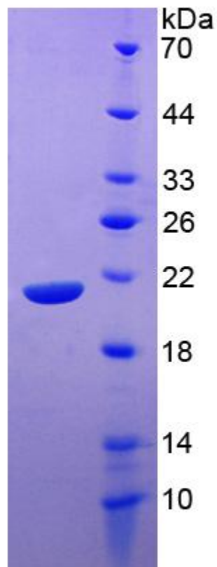
15% SDS-PAGE
