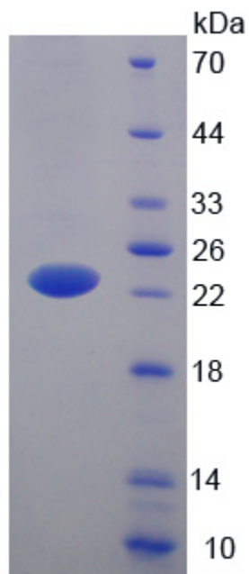
15% SDS-PAGE
