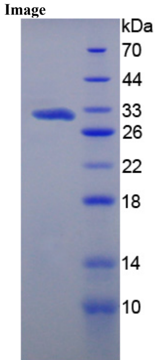
15% SDS-PAGE
